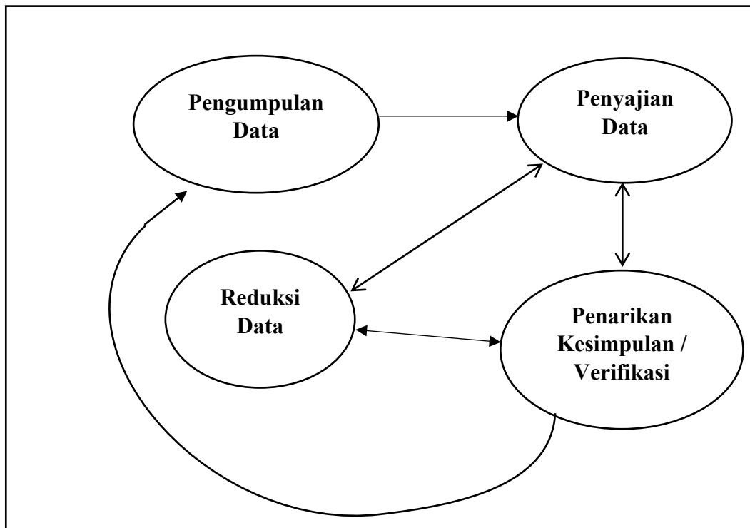
Gambar 3.1 Analisis Data model interaktif Miles dan Huberman
